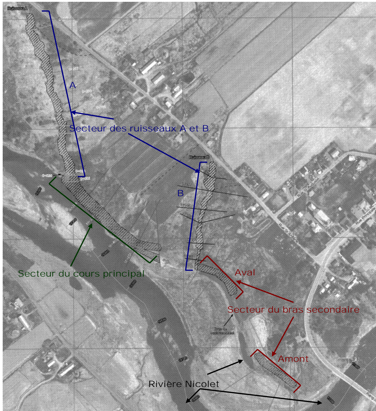
FIGURE 2 : VUE EN PLAN DES TROIS SECTEURS DES TRAVAUX DE STABILISATION DES TALUS
